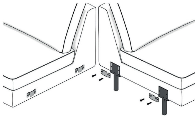
Montage Universalstützfüße
